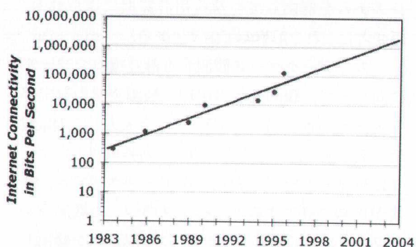
図3 Nielsen の法則。横軸は年（西暦）である。
