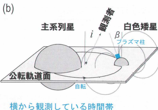
図3 b 磁極にあるX線放射領域と我々の視線方向の関係。
