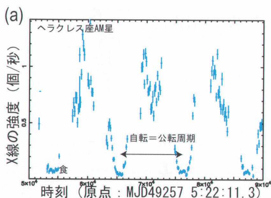
図3 a ポーラーの代表格、ヘラクレースAM星のX線ライトカーブ。「あすか」による観測。
