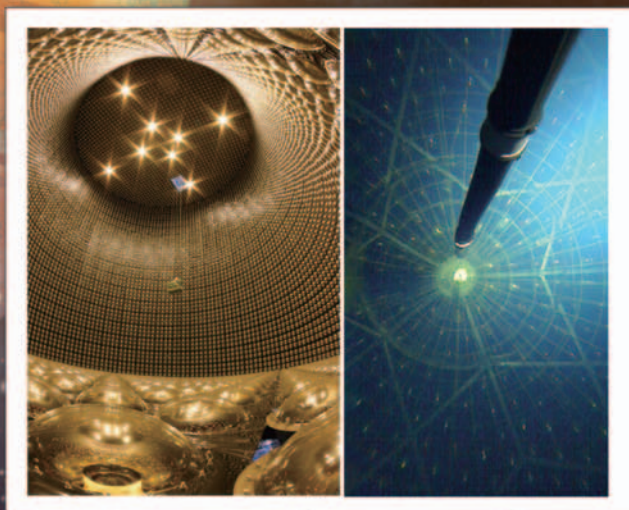
(左) スーパーカミオカンデ検出器内部の様子 (右) カムランド検出器内部の様子
