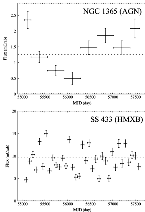
図3. 軟X線(4-10 keV)の光度曲線の例. 横軸は修正ユリウス日, 縦軸は「かに星雲」の1000分1のX線フラックスに対する相対強度を表している. 破線は各々の天体の7年平均光度である. (上) AGN(セイファートI型銀河)であるNGC 1365の1年単位の光度曲線. ただし, 最初と最後の2009年と2016年のピンは, 約5ヶ月と7ヶ月の平均値に相当する. (下) 大質量X線連星系(HMXB: High-Mass X-ray Binary)であるSS 433の73日単位の光度曲線.
