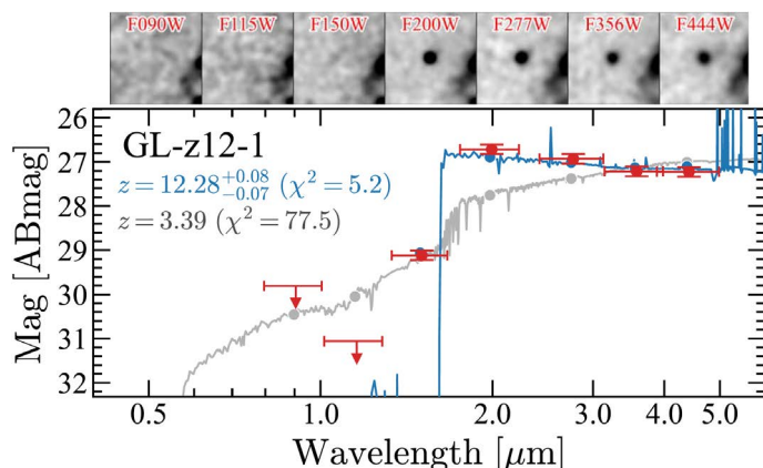
図3 JWSTの初期データから見つけた明るい z \sim 12 銀河候補GL-z12-1[26]。上パネルはJWST/NIRCamの画像を示している。F150Wバンドを境に長波長側では明るく、短波長側では暗くなっており、画像だけでもF150W-ドロップアウト銀河であることがはっきりとわかる。下パネルは丸印が観測された各バンドごとの等級（スペクトルエネルギー分布；SED）を示しており、 z \sim 12 銀河のモデル（青線）とよく合うことがわかる。この銀河はのちのNIRSpec分光観測で、赤方偏移が z = 12.34 であることが確認されている [27]。
