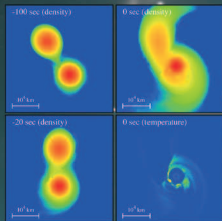
二重白色矮星の合体シミュレーション
