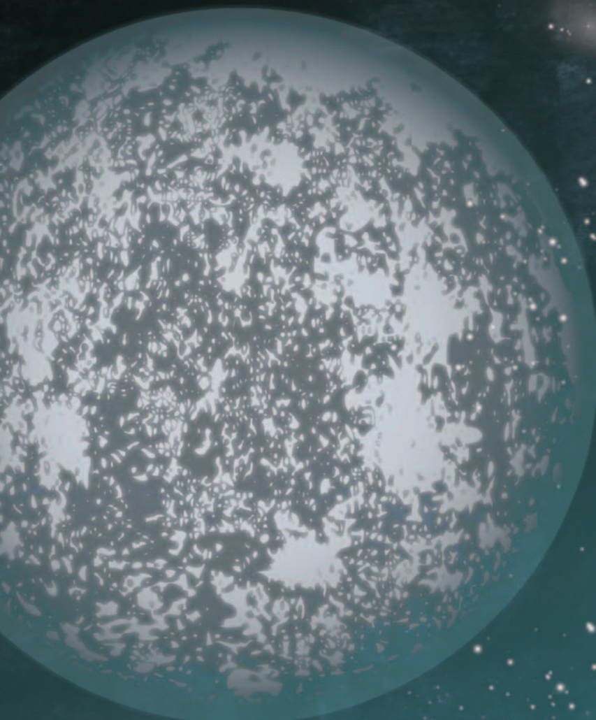
二重白色矮星の合体シミュレーション
