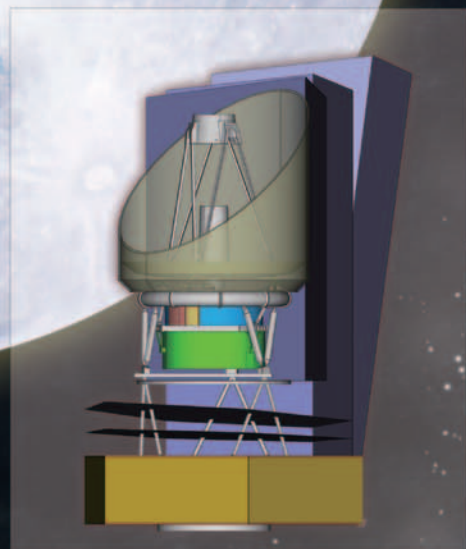
次世代赤外線天文衛星 SPICA の最新構成図(ESA提供)
