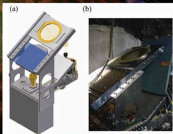
Z45の設計段階の概略図と野辺山45m鏡に搭載したZ45の現物写真
