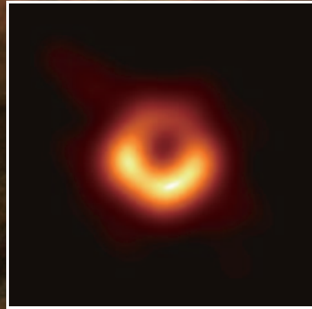
EHTによって撮影された 超巨大ブラックホールM87*
