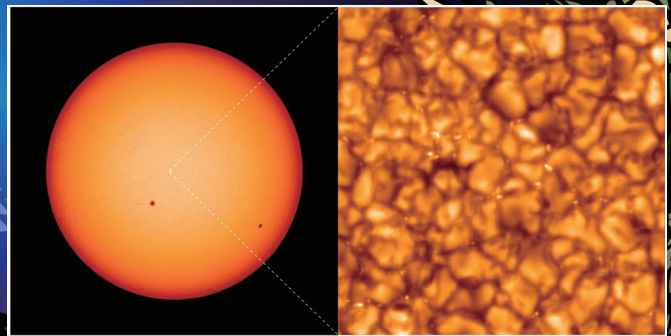
科学衛星「ひので」 可視光磁場望遠鏡が捉えた太陽表面
