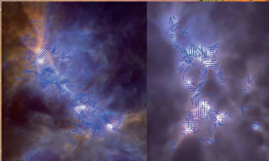
BISTRO の観測した星形成領域内部の複雑な磁場構造
