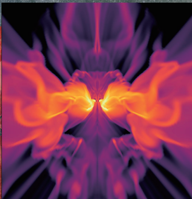
初代銀河の中心核で急成長する種ブラックホールの様子
