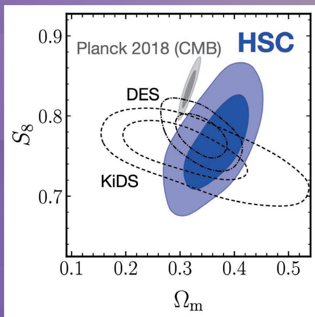
HSC Y3 の 3x2pt 解析結果と他の宇宙論観測の結果の比較
