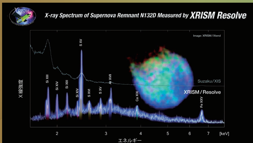
XRISM ファーストライト観測 (超新星残骸 N132D)
