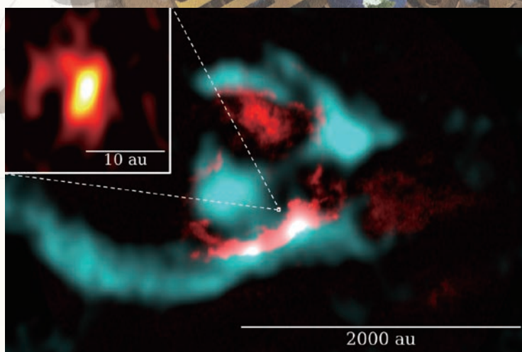
MC27分子雲コアのALMA観測
