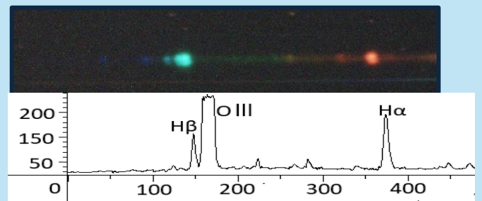
↑ 図2 NGC 7027 実直径 16,560au
