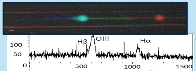
↑ 図1 まばたき星雲 実直径 84,600au
