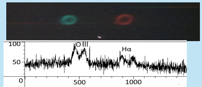
↑ 図3 M57 実直径 119,550au
